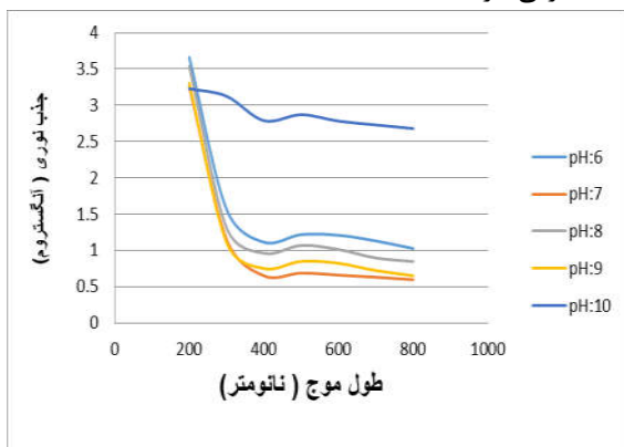
نمودار ۱. طیف اسپکتروفوتومتری فرابنفش-مرئی نانوذرات نقره سنتز شده در pH های متفاوت (۶، ۷، ۸، ۹ و ۱۰).
