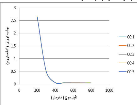
نمودار ۲. طیف اسپکتروفوتومتری فرابنفش-مرئی نانوذرات نقره سنتز شده به کمک غلظت های ۱، ۲، ۳، ۴ و ۵ میلی مولار از عصاره گیاه خرفه.
